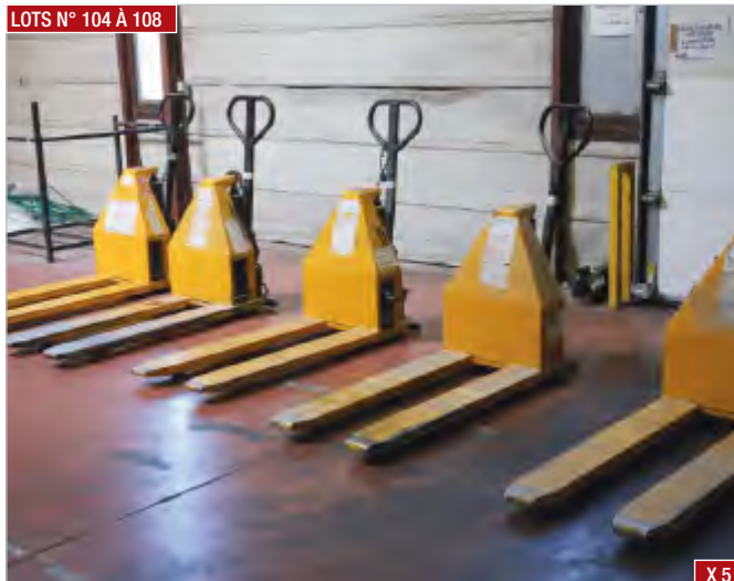
► Transpalettes électrique MIC , type TMXE1000, cap 1 T, Ht de levée 800 mm ► MIC electric pallet jack, type TMXE 1000, lifting height 800 mm, max 1T
